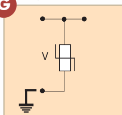
G 2-полюсная варисторная защита
