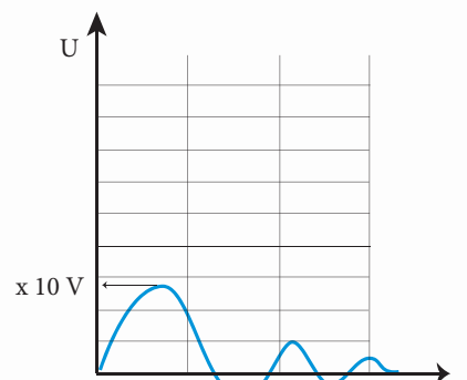
Четвертьволновой разрядник
