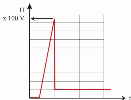
Газовый разрядник
