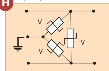
H 3-полюсная варисторная защита
